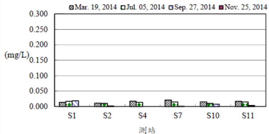
圖11、103年後灣附近海域各測站氨氮之變化
