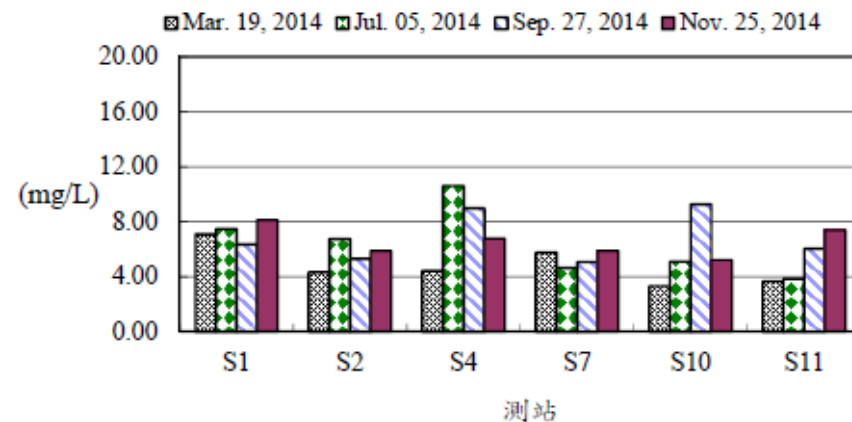
圖14、103年後灣附近海域各測站海水中懸浮固體量之變
