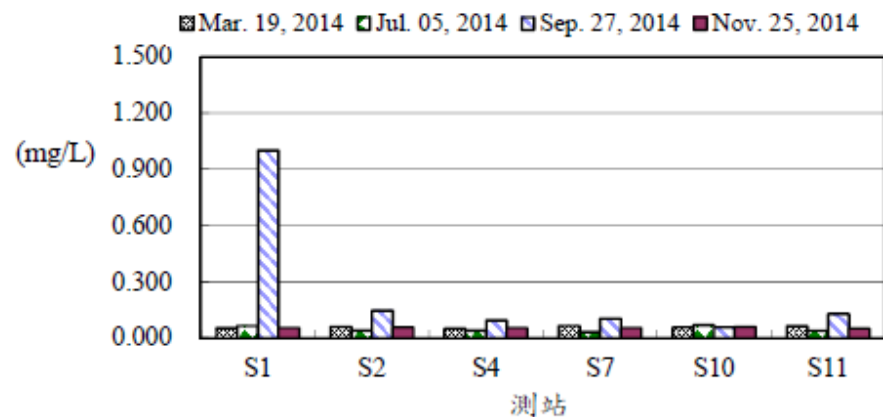
圖10、103年後灣附近海域各測站矽酸鹽之變化
