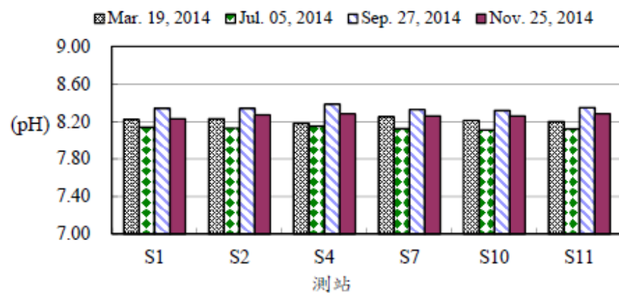
圖5、103年後灣附近海域各測站海水pH之變化
