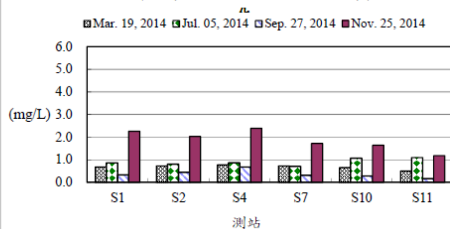
圖6、103年後灣附近海域各測站五天生化需氧量之變
