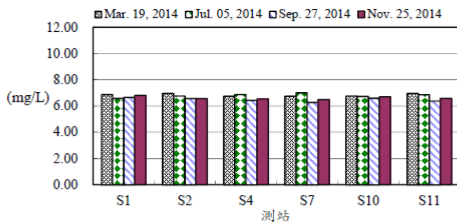
圖4、103年後灣附近海域各測站海水溶氧量之變化
