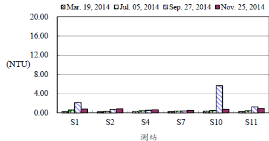
圖12、103年後灣附近海域各測站海水濁度之變化
