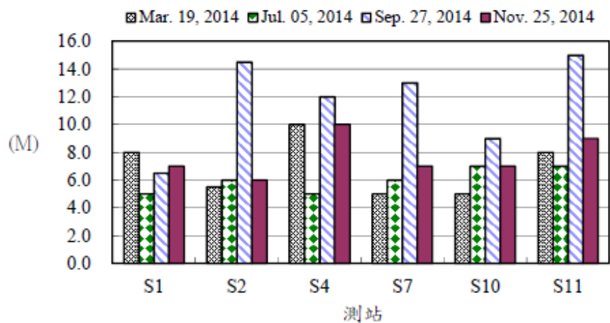
圖1、103年後灣附近海域各測站透視度之變化
