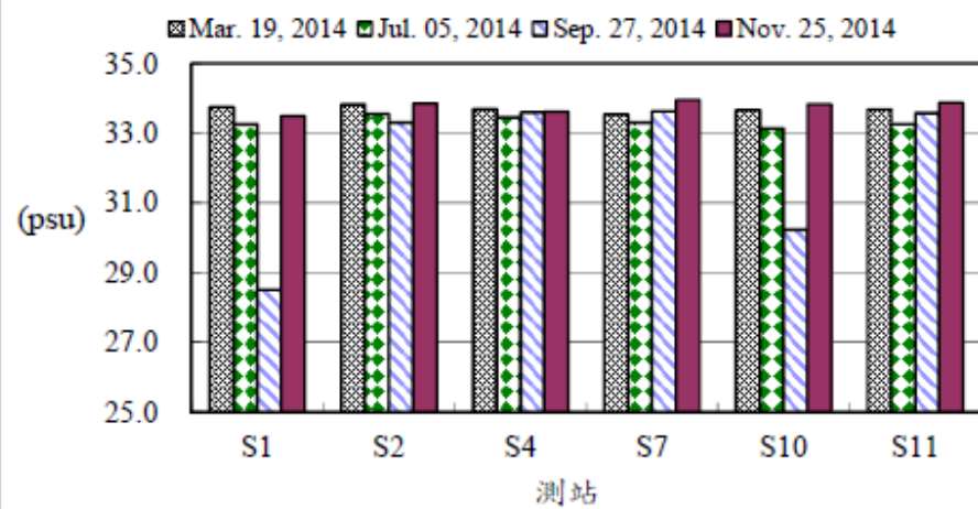
圖2、103年後灣附近海域各測站海水鹽度之變化
