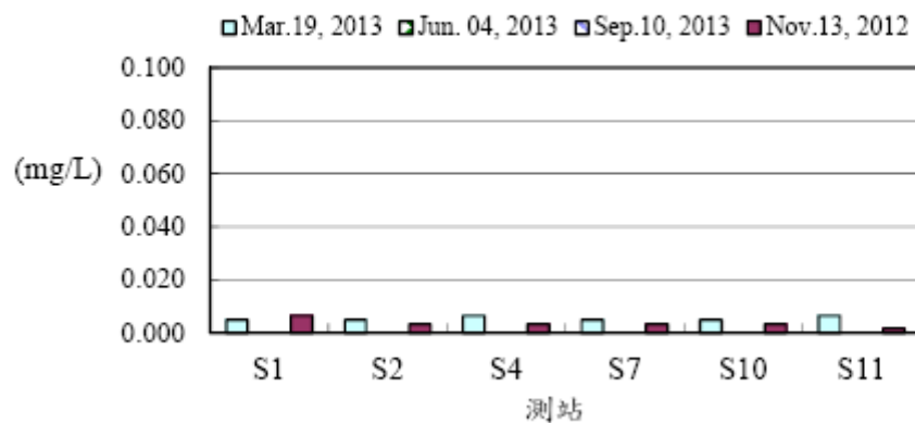
圖9、102年後灣附近海域各測站磷酸鹽之變化
