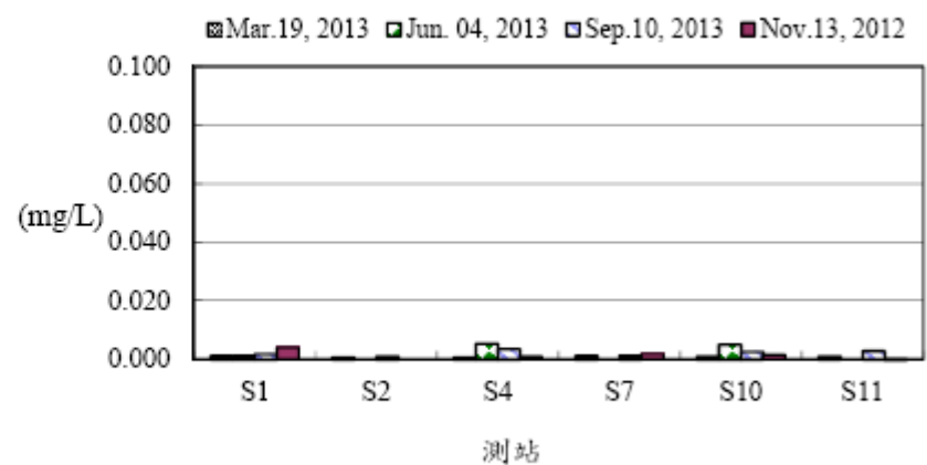
圖8、102年後灣附近海域各測站亞硝酸鹽之變化
