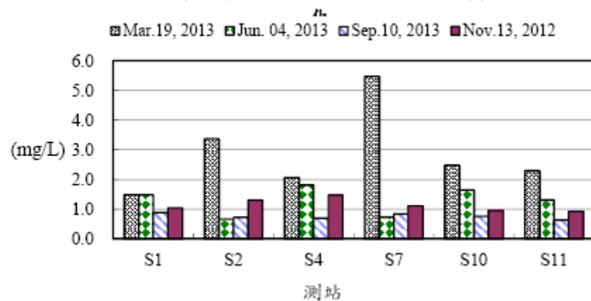
圖6、102年後灣附近海域各測站五天生化需氧量之變
