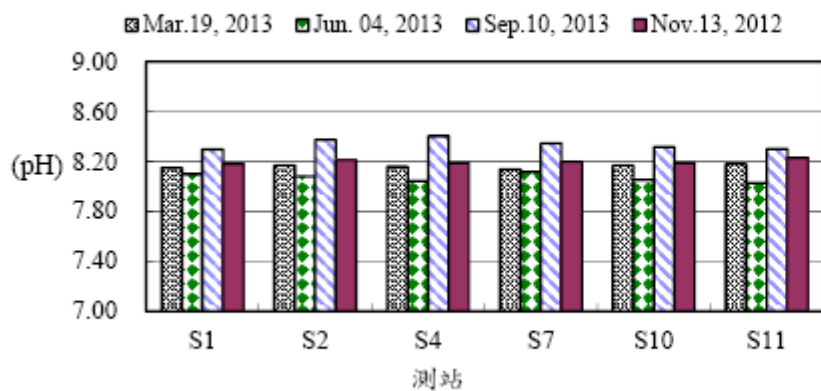
圖5、102年後灣附近海域各測站海水pH之變化
