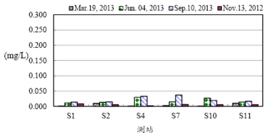
圖11、102年後灣附近海域各測站氨氮之變化
