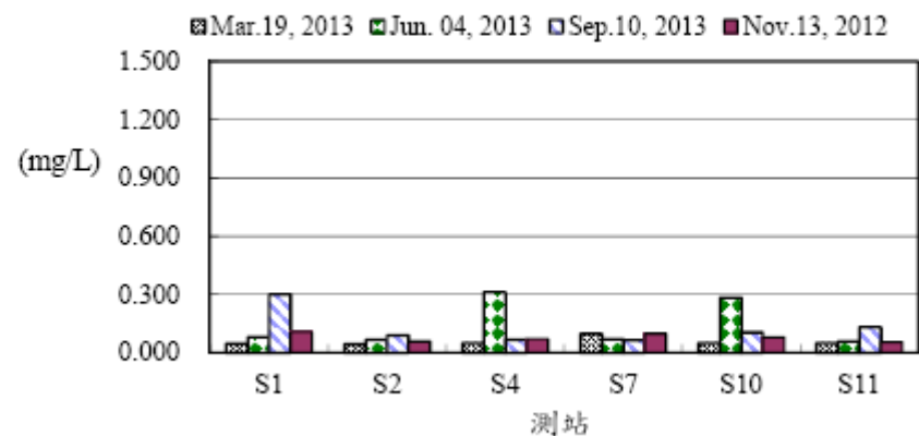
圖10、102年後灣附近海域各測站矽酸鹽之變化
