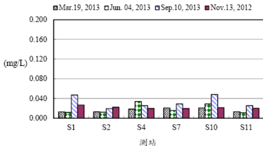
圖7、102年後灣附近海域各測站硝酸鹽之變化
