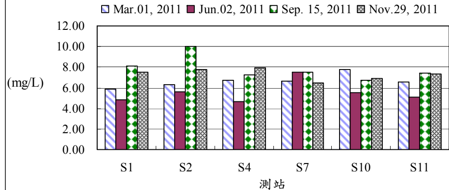
圖4、100年後灣附近海域各測站海水溶氧量之變化
