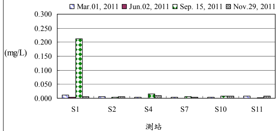
圖11、100年後灣附近海域各測站氨氮之變化
