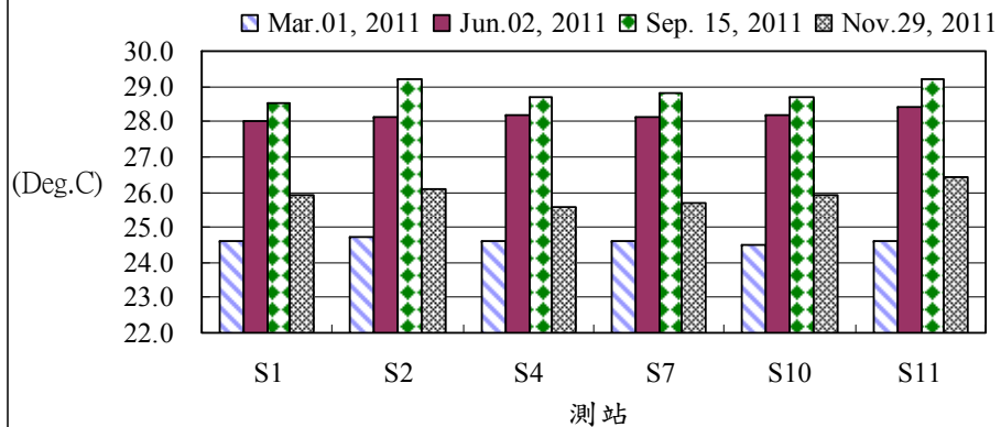
圖3、100年後灣附近海域各測站海水溫度之變化
