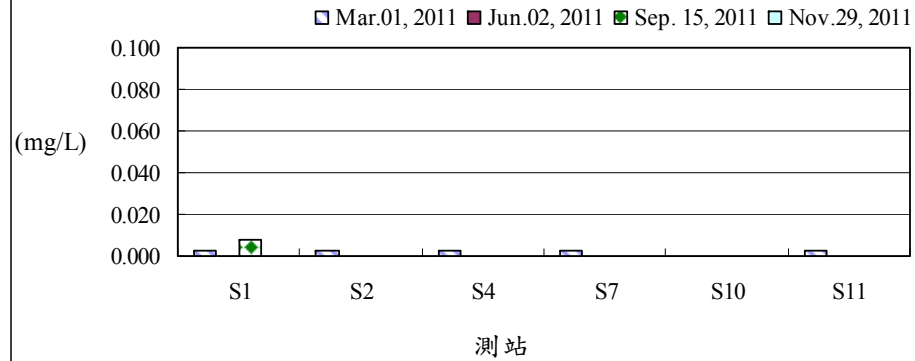
圖9、100年後灣附近海域各測站磷酸鹽之變化
