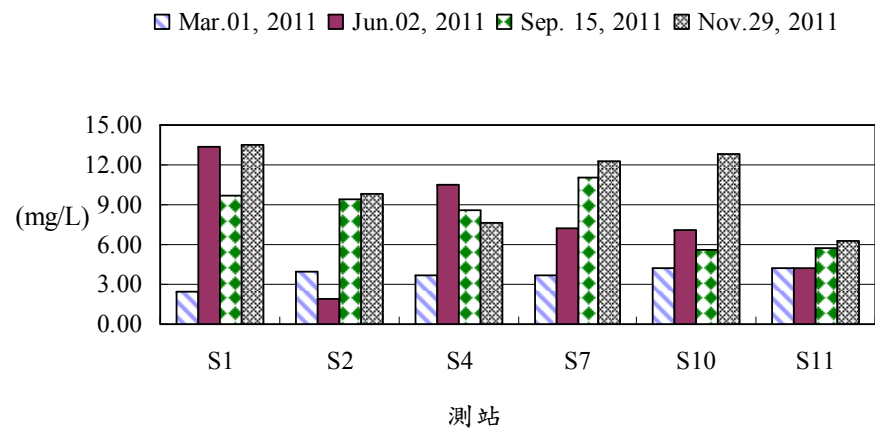
圖 14、100年後灣附近海域各測站海水中懸浮固體量之變化
