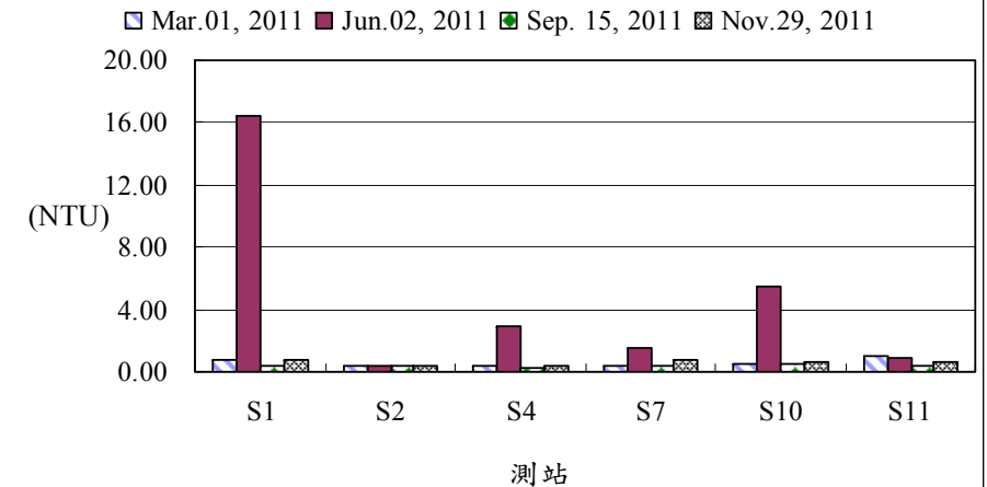
圖12、100年後灣附近海域各測站海水濁度之變化
