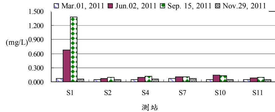
圖10、100年後灣附近海域各測站矽酸鹽之變化
