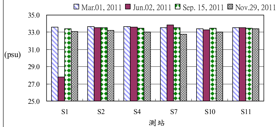
圖2、100年後灣附近海域各測站海水鹽度之變化
