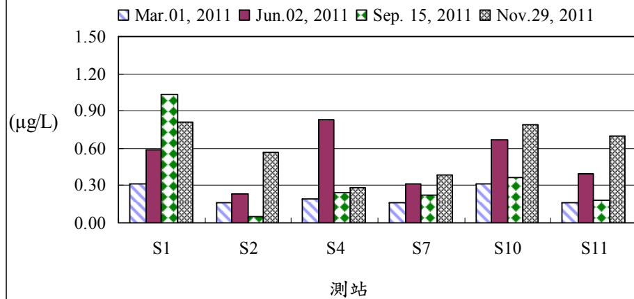
圖 13、100年後灣附近海域各測站葉綠素甲量之變化
