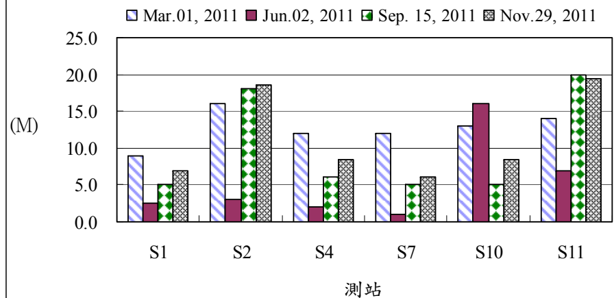
圖1、100年後灣附近海域各測站透視度之變化
