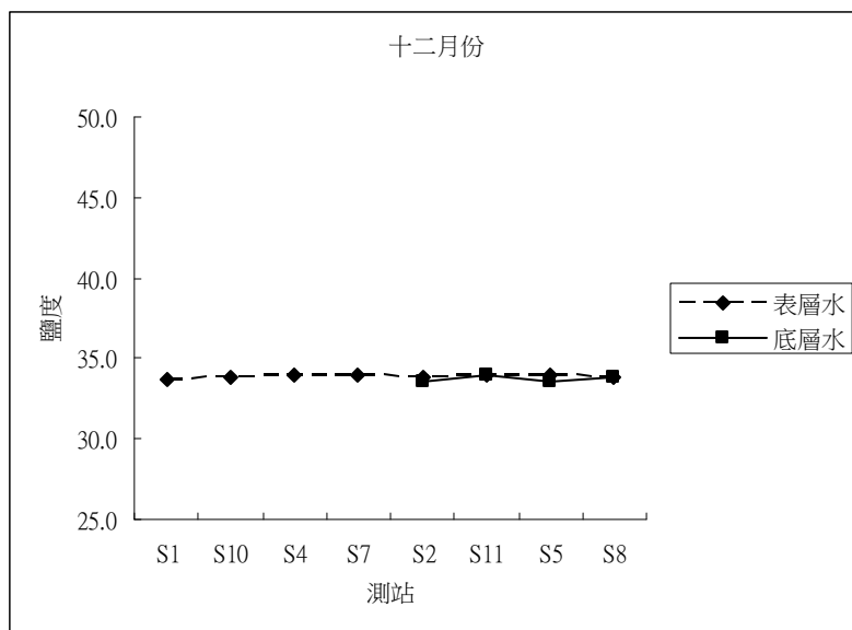
圖 5 後灣附近海域 98 年 2、5、6、8、10、12 月海水鹽度之變化
