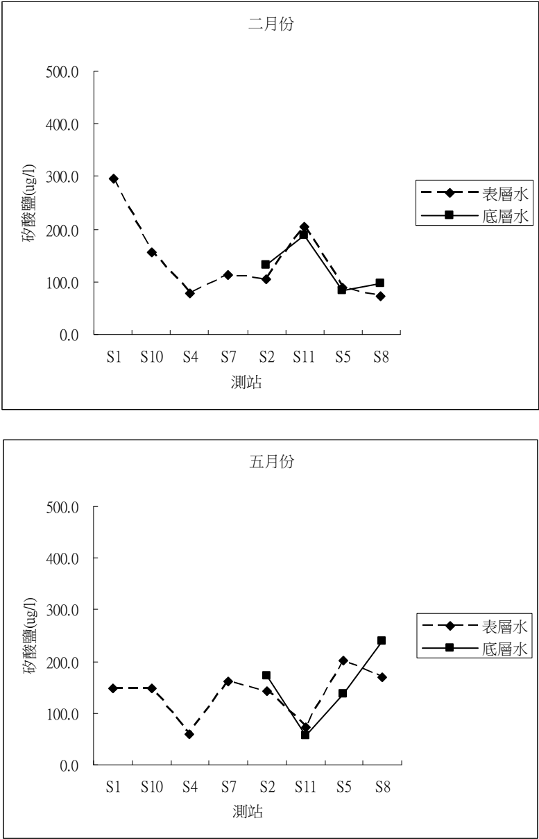
圖 10 後灣附近海域 98 年 2、5、6、8、10、12 月海水硝酸鹽之變化
