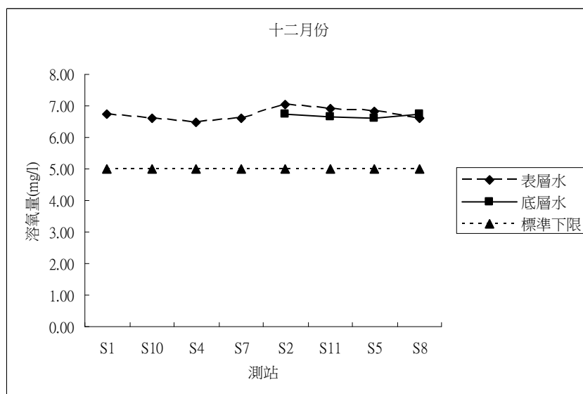
圖 3 後灣附近海域 98 年 2、5、6、8、10、12 月海水溶氧量之變化
