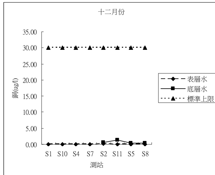
圖 18 後灣附近海域 98 年 2、5、6、8、10、12 月海水銅含量之變化
