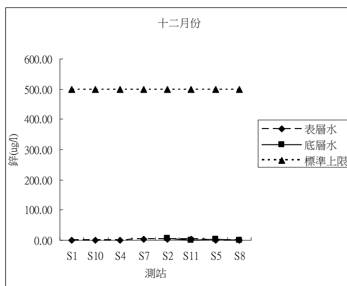
圖 17 後灣附近海域 98 年 2、5、6、8、10、12 月海水鉅含量之變化
