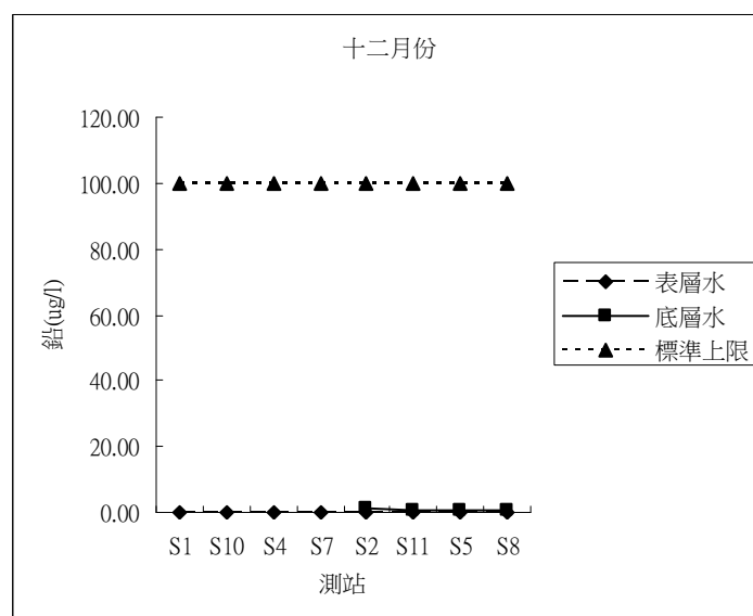
圖 16 後灣附近海域 98 年 2、5、6、8、10、12 月海水鉛含量之變化
