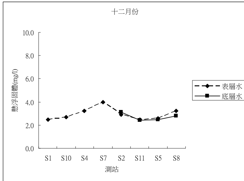
圖 6 後灣附近海域 98 年 2、5、6、8、10、12 月海水懸浮固體之變化
