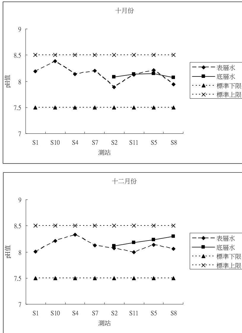
圖 1 後灣附近海域 98 年 2、5、6、8、10、12 月海水 pH 值之變化
