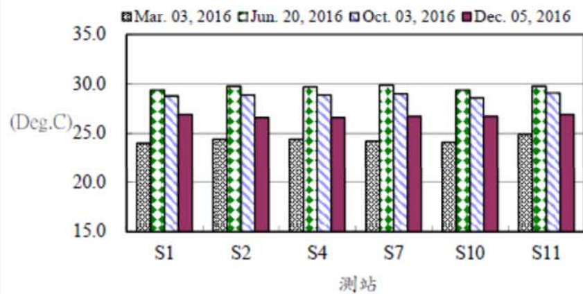
圖3、105年後灣附近海域各測站海水溫度之變化
