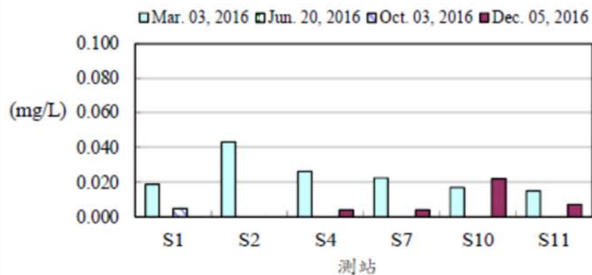
圖9、105年後灣附近海域各測站磷酸鹽之變化
