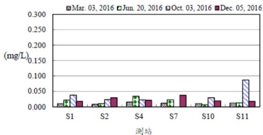
圖11、105年後灣附近海域各測站氨氮之變化
