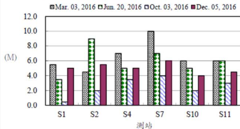
圖1、105年後灣附近海域各測站透視度之變化
