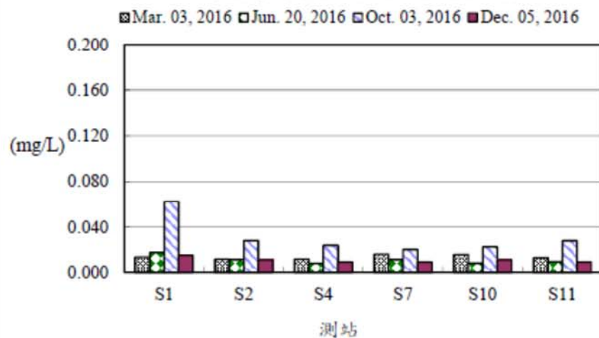
圖7、105年後灣附近海域各測站硝酸鹽之變化
