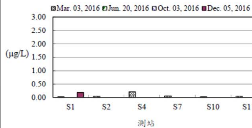
圖13、105年後灣附近海域各測站葉綠素甲量之變化
