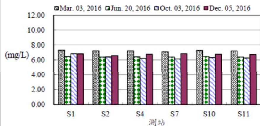
圖4、105年後灣附近海域各測站海水溶氧量之變化
