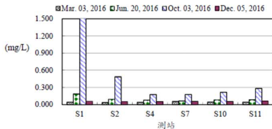
圖10、105年後灣附近海域各測站矽酸鹽之變化
