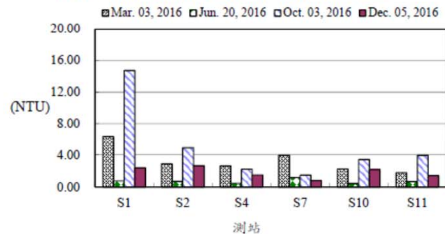
圖12、105年後灣附近海域各測站海水濁度之變化
