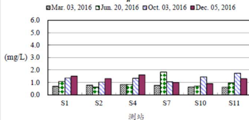
圖6、105年後灣附近海域各測站五天生化需氧量之變
