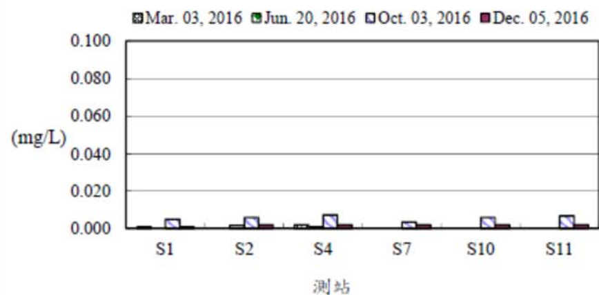
圖8、105年後灣附近海域各測站亞硝酸鹽之變化
