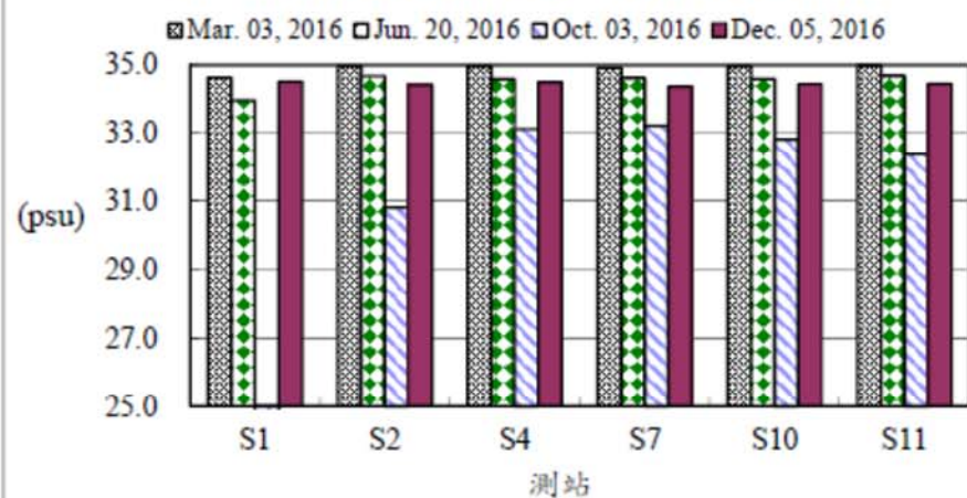
圖2、105年後灣附近海域各測站海水鹽度之變化
