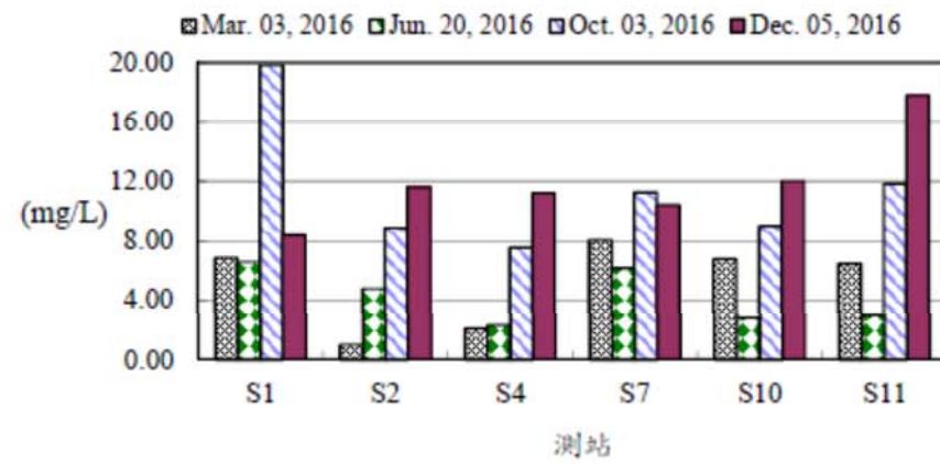
圖14、105年後灣附近海域各測站海水中懸浮固體量之變化
