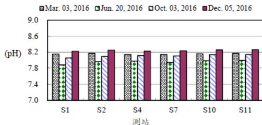
圖5、105年後灣附近海域各測站海水pH之變化
