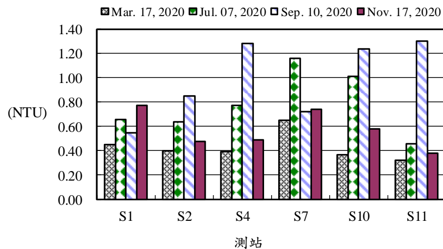
圖12、109年後灣附近海域各測站海水濁度之變化
