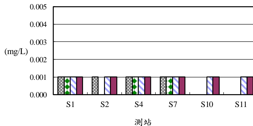
圖8、109年後灣附近海域各測站亞硝酸鹽之變化
