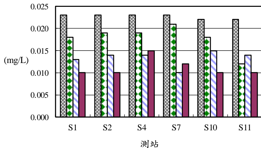
圖7、109年後灣附近海域各測站硝酸鹽之變化
