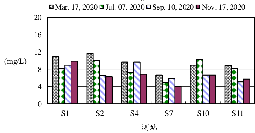
圖14、109年後灣附近海域各測站海水中懸浮固體量之變
