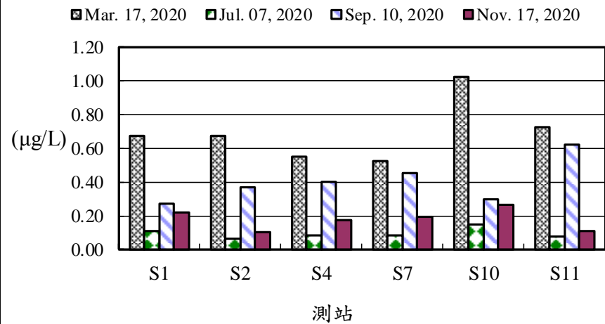
圖13、109年後灣附近海域各測站葉綠素甲量之變化
