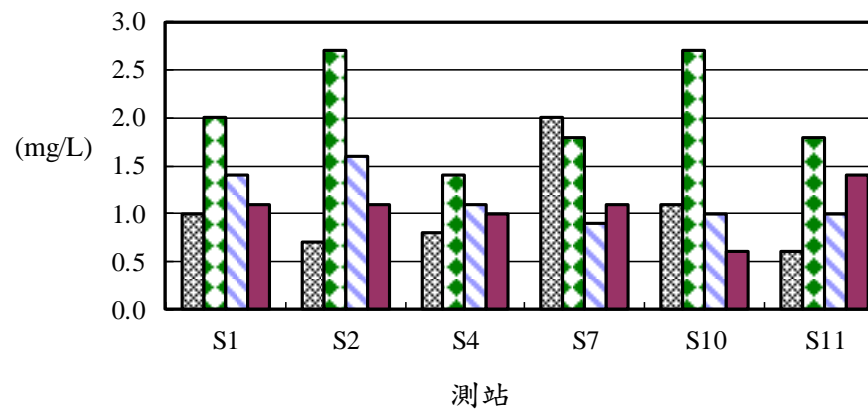
圖8、109年後灣附近海域各測站亞硝酸鹽之變化
