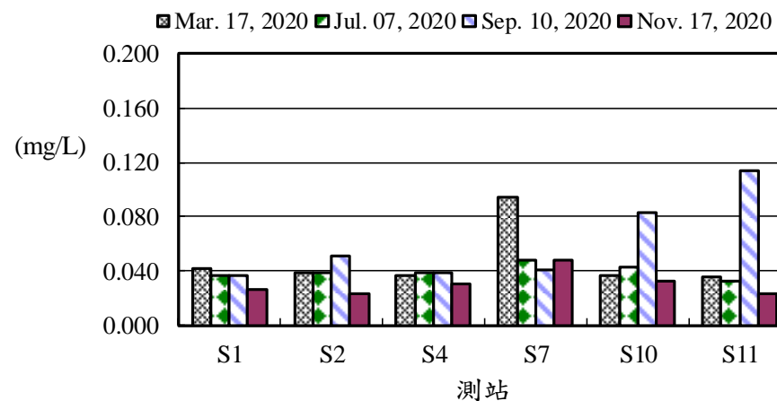
圖10、109年後灣附近海域各測站矽酸鹽之變化
