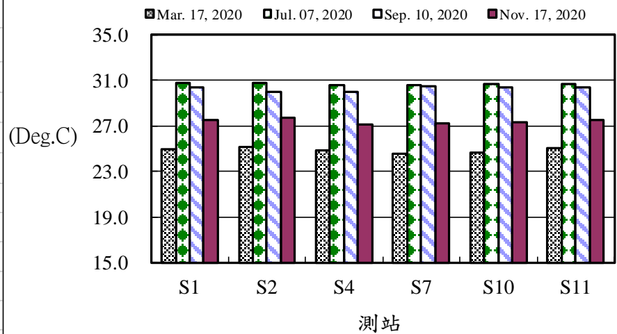
圖3、109年後灣附近海域各測站海水溫度之變化
