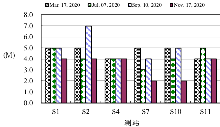
圖1、109年後灣附近海域各測站透明度之變化
