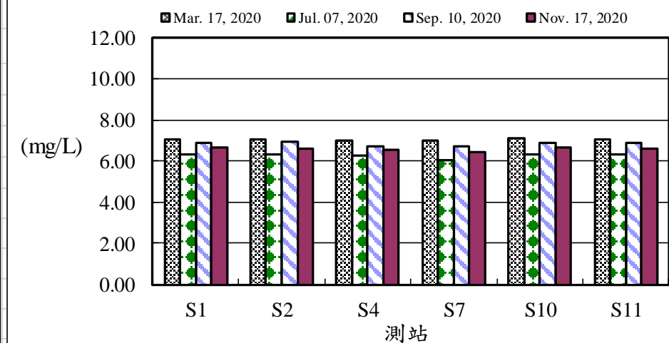
圖4、109年後灣附近海域各測站海水溶氧量之變化
