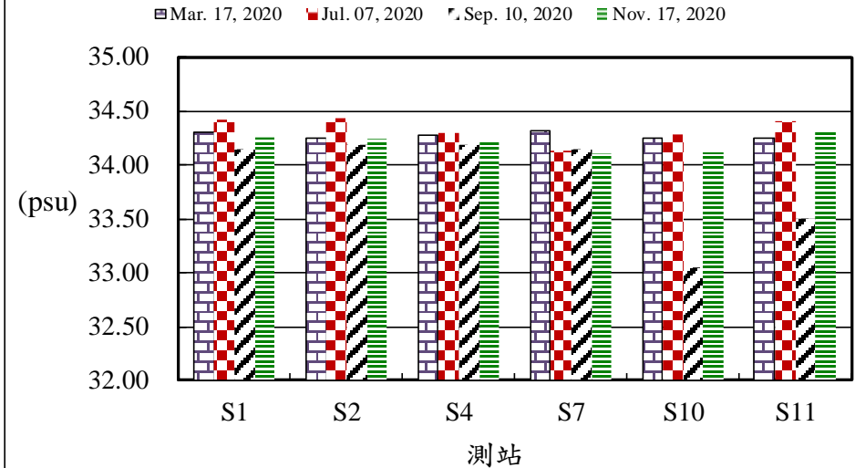
圖2、109年後灣附近海域各測站海水鹽度之變化
