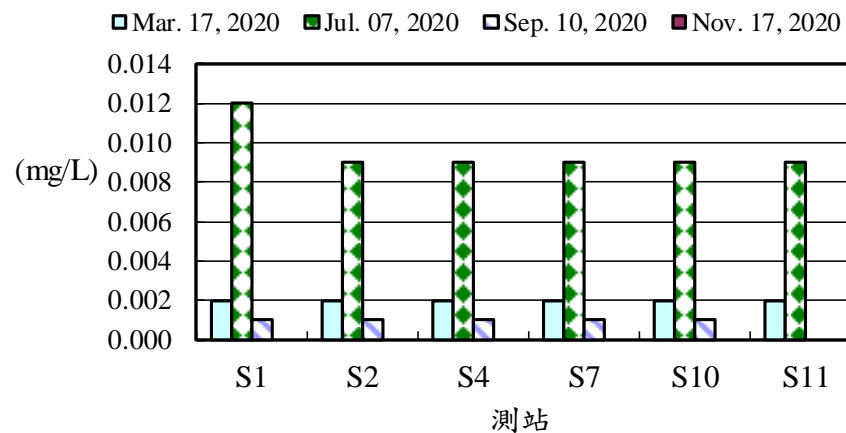
圖9、109年後灣附近海域各測站正磷酸鹽之變化
