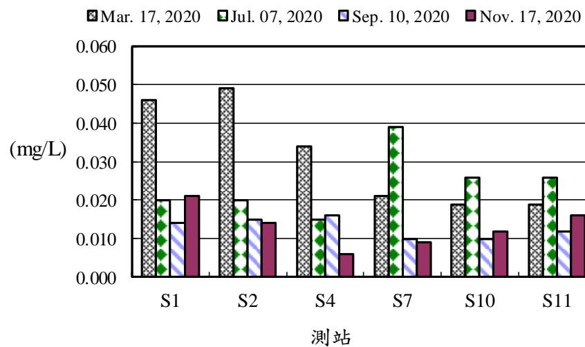
圖11、109年後灣附近海域各測站氨氮之變化
